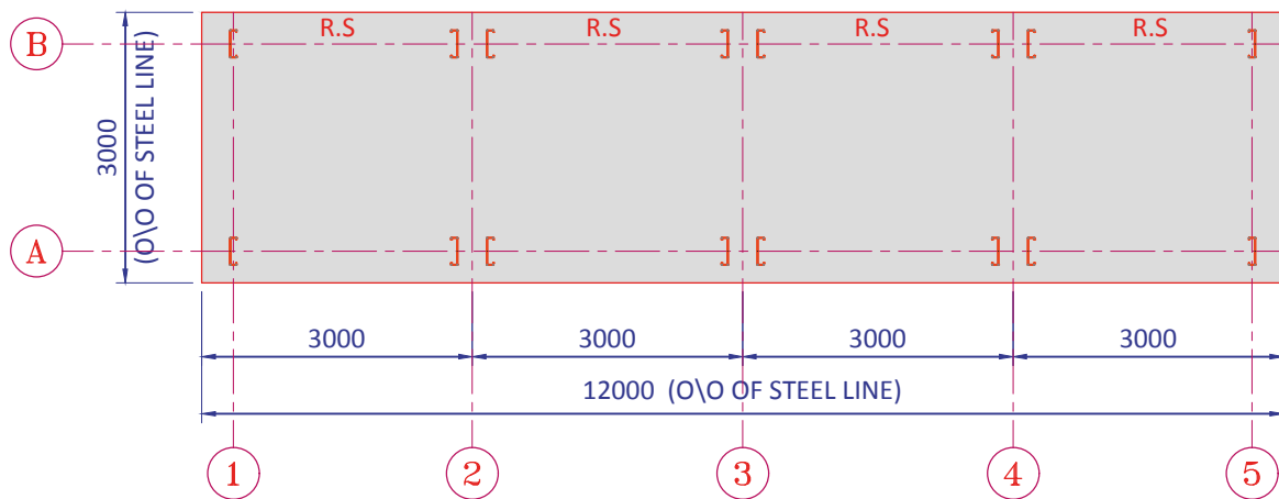
FLOOR PLAN 3x12x3M KIOSKS
